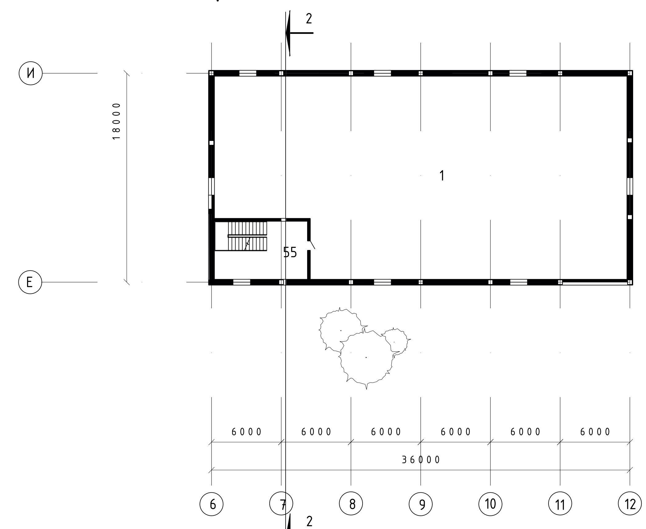
План четвертого этажа АБК 1:200
