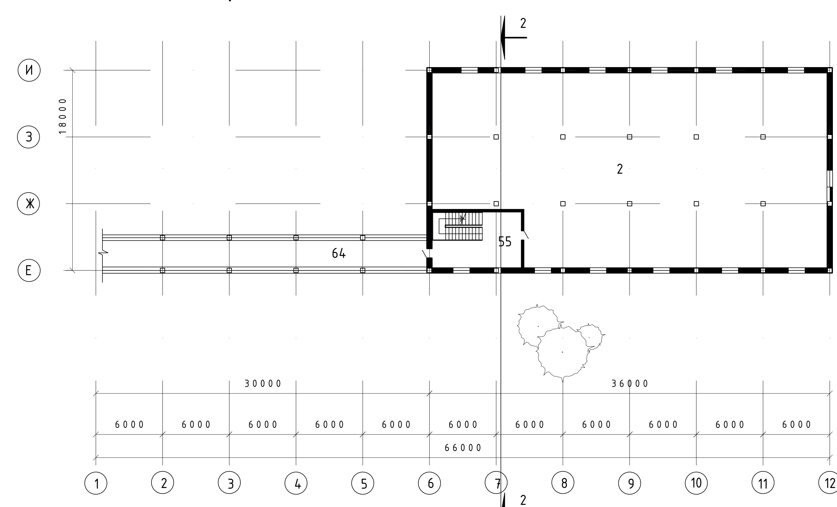
План третьего этажа АБК 1:200
