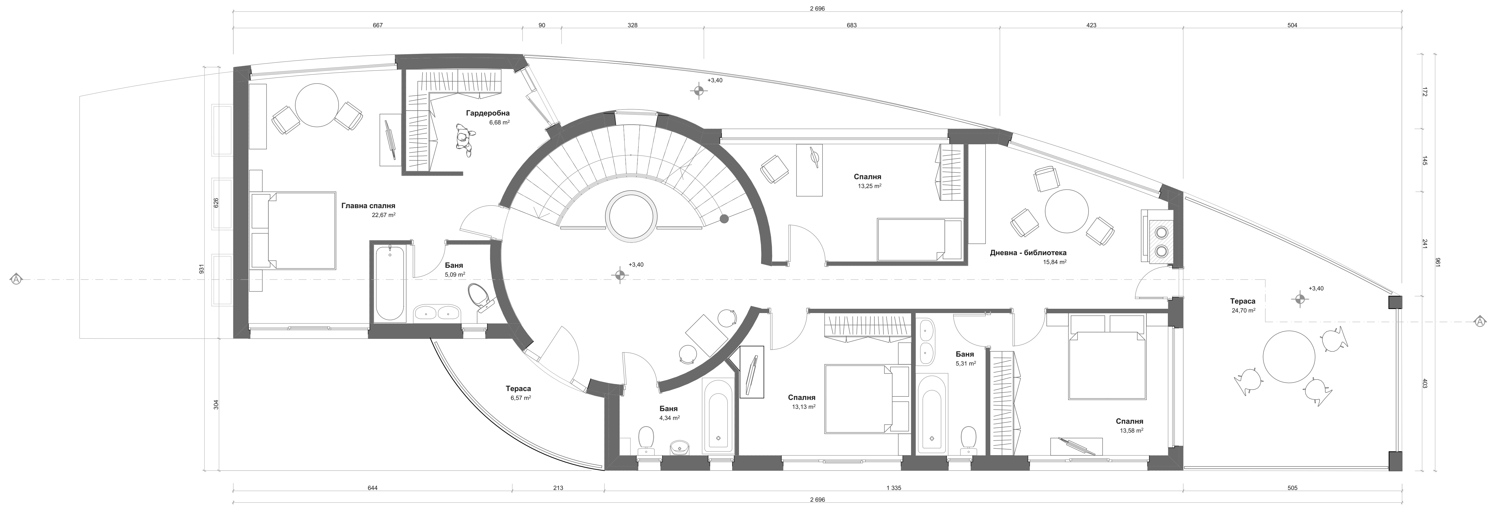
ПЛАН ЕТАЖ 2 КОТА +3.40 М1:50
