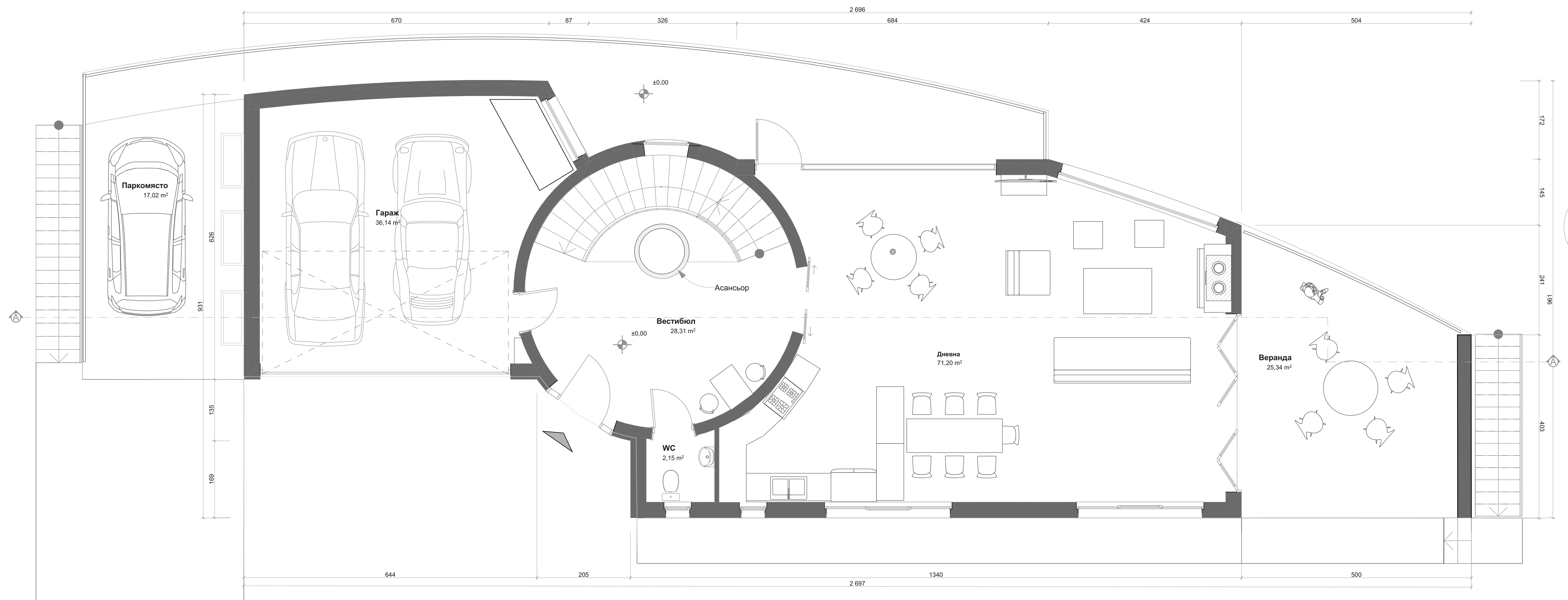
ПЛАН ЕТАЖ 1 КОТА ±0.00 М1:50
